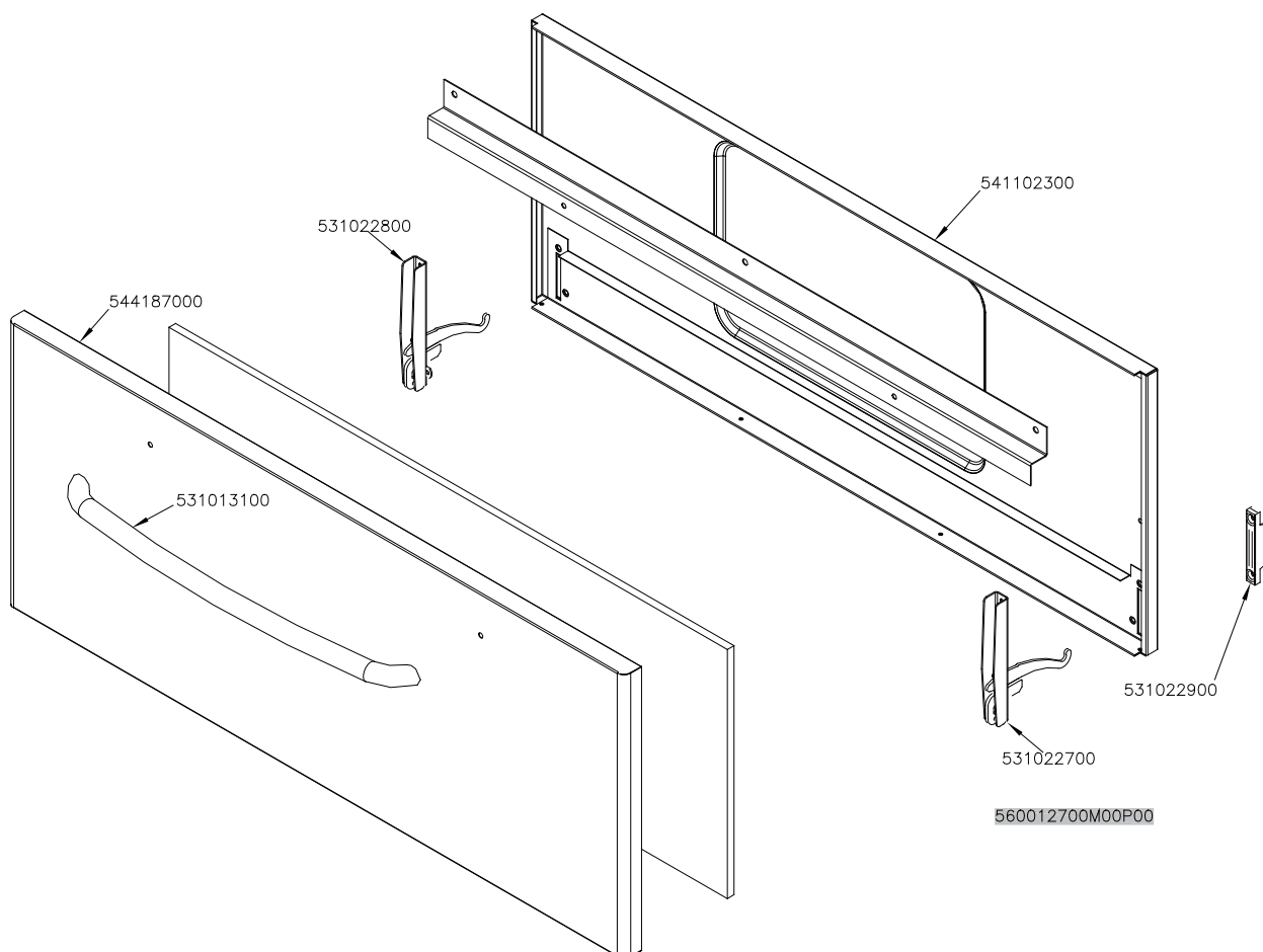
GN 3/1
