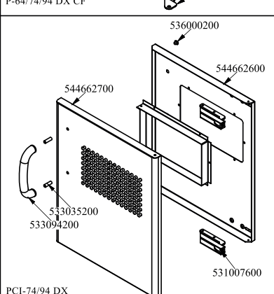
PCI-74/94 DX
