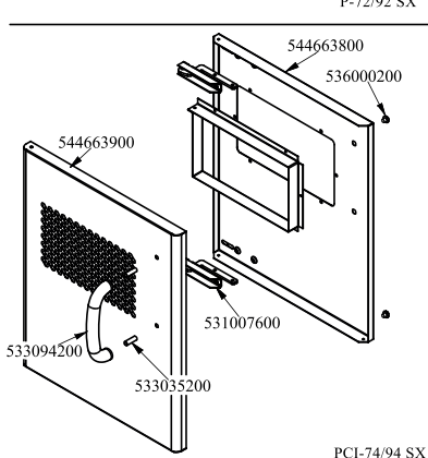
PCI-74/94 SX
